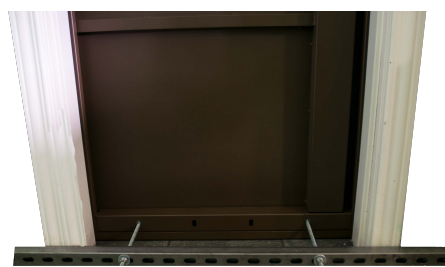
ANCLAJE PARED SUPERIOR E INFERIOR
